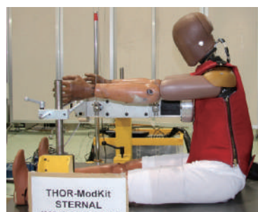
次世代前面衝突用人体ダミーに対する衝撃試験 Evaluation test for advanced frontal impact dummy
