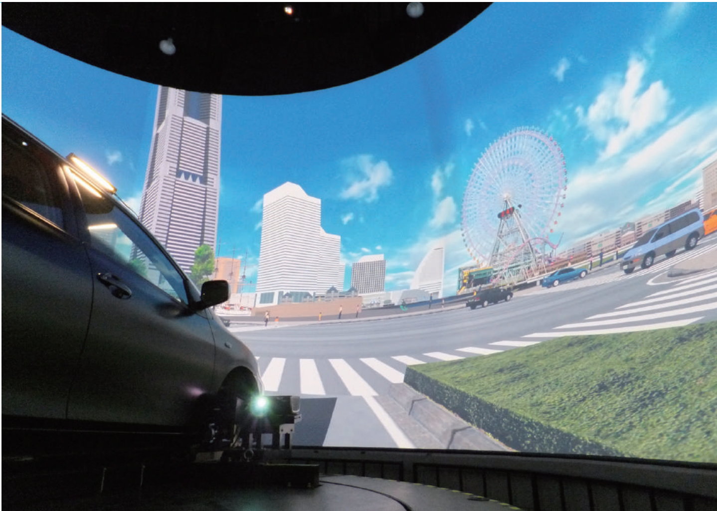
全方位視野ドライビングシミュレータ実験風景(市街地) Omni-directional viewing driving simulator test (city area)
