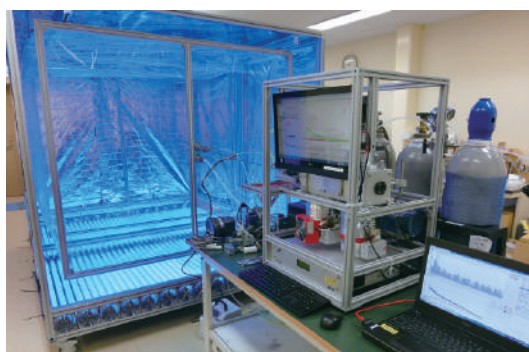
光化学スモッグチャンバー反応装置 (PM 2.5 二次生成のメカニズム解明に向けた研究) Photochemical smog chamber reactor (Research for studying the mechanisms of secondary generation of PM 2.5 )
