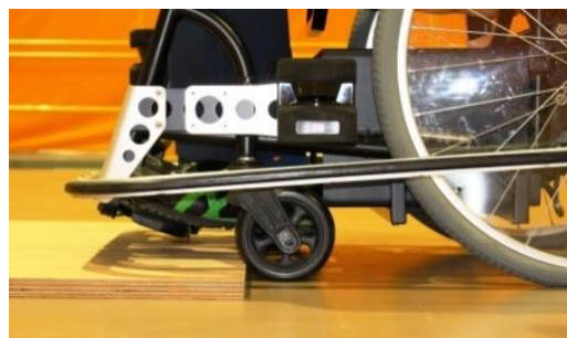
段差乗り越え試験
