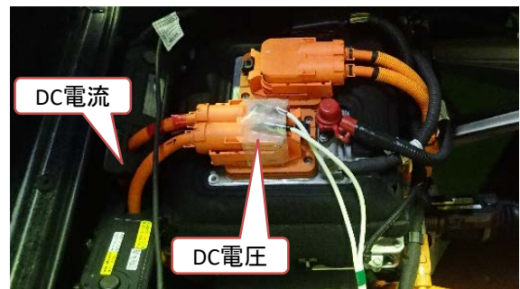
駆動用バッテリーの電圧／電流測定
