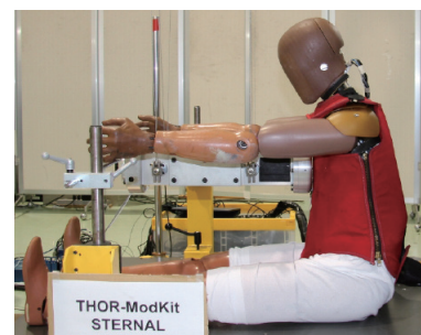
次世代前面衝突用人体ダミーに対する衝撃試験 Evaluation test for advanced frontal impact dummy
