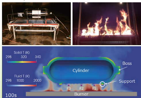
高圧容器の火災暴露試験(上)と火災暴露試験数値シミュレーション(下) Flame exposure test on high-pressure vessel (top). Flame exposure test value simulation (bottom).
