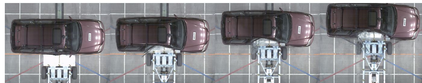
ムービングデフォーマルバリアによる側面衝突試験 Side collision test using moving deformable barrier
