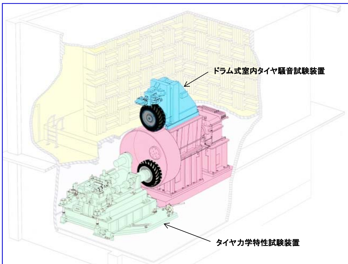
タイヤ力学特性試験装置およびドラム式室内タイヤ騒音試験装置
