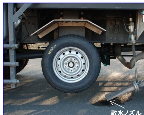
路上タイヤ試験車測定輪 (右前輪と右後輪の間に装備)
